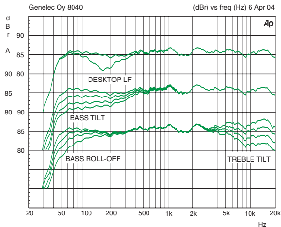
Kuva 7. "Bass tilt"- , "treble tilt"- , "desktop low frequency"- ja "bass roll-off"-säätöjen vaikutus 8040B:n vapaakenttävasteeeseen.
