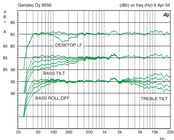
Kuva 9. "Bass tilt"- , "treble tilt"- , "desktop low frequency"- ja "bass roll-off"-säätöjen vaikutus 8050B:n vapaakenttävasteeeseen.
